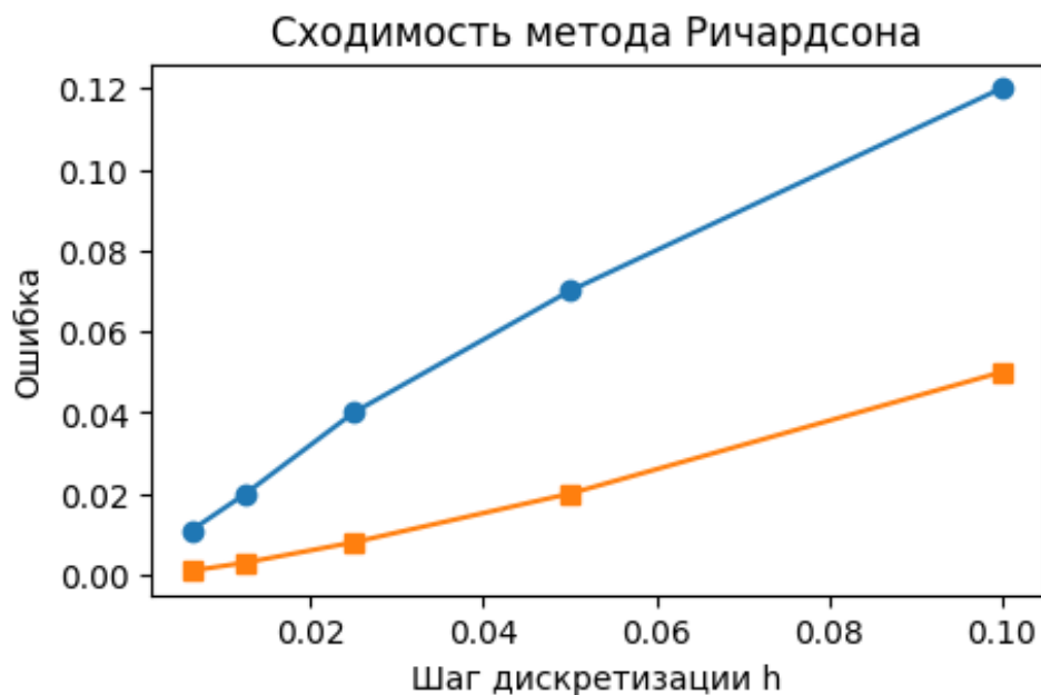
Рис. 1. Сходимость метода экстраполяции Ричардсона при уменьшении шага дискретизации
