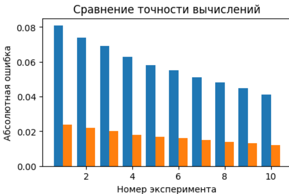
Рис. 2. Сравнение точности вычислений с экстраполяцией и без методов Ричардсона
