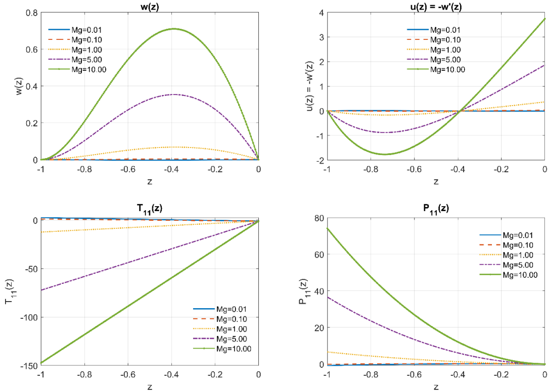
Рис. 1. Профили w(z) , u(z) = -w'(z) , T_{11}(z) и P_{11}(z) для Mg = 0.01, 0.1, 1, 5, 10
