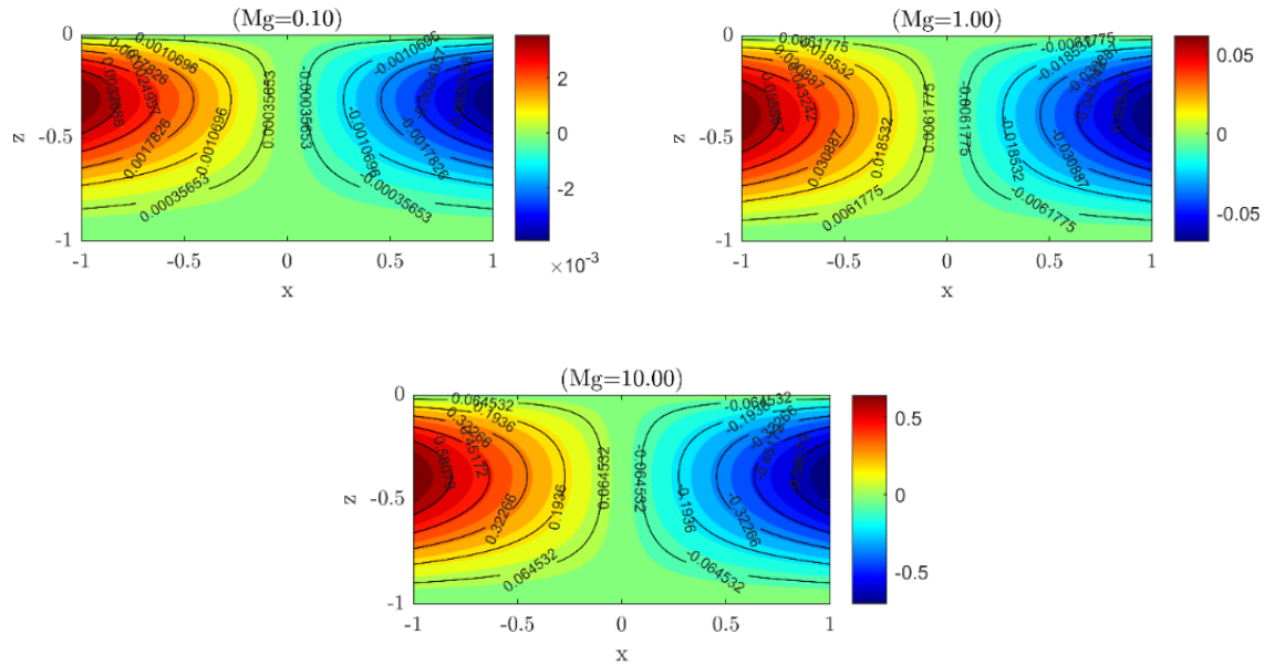
Рис. 2. Изолинии функции тока \psi(x, z) для Mg = 0.1, 1, 10
