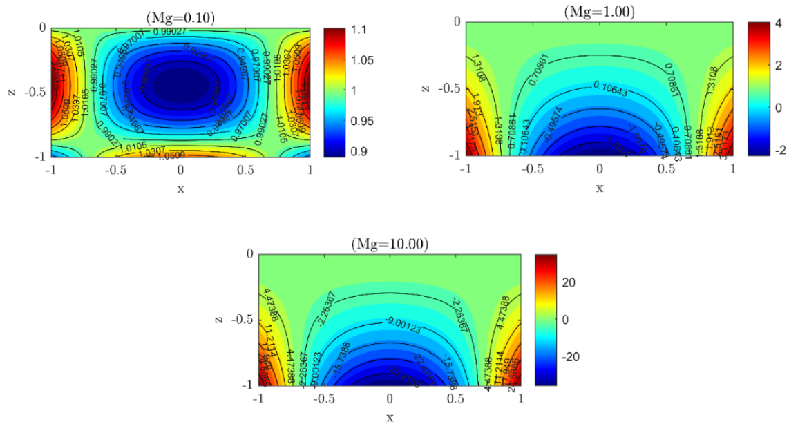
Рис. 3. Изолинии давления P(x, z) для Mg = 0.1, 1, 10
