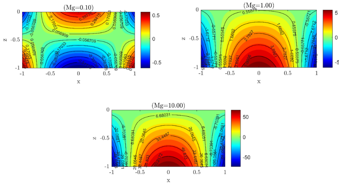
Рис. 4. Изолинии температуры T(x, z) для Mg = 0.1, 1, 10
