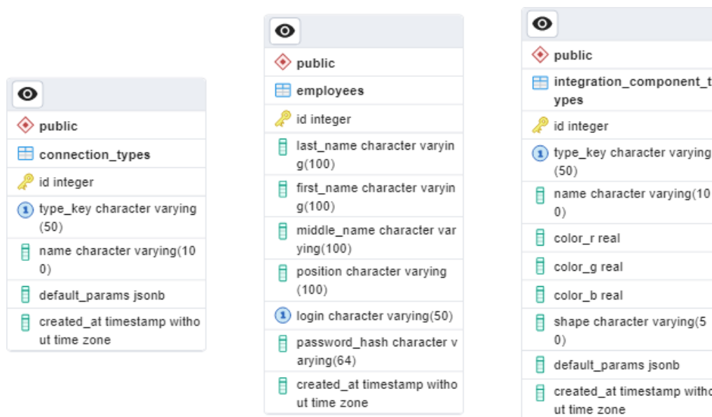
Рис. 7. Физическая схема базы данных
