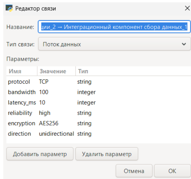
Рис. 4. Диалог редактирования связи: тип, протокол и параметры взаимодействия
