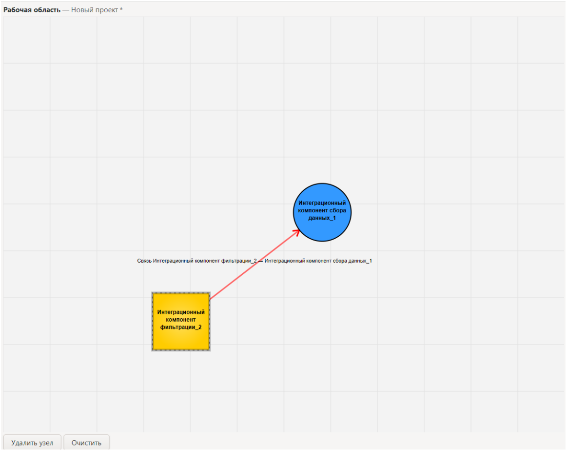
Рис. 3. Пример связи «Поток данных» между двумя интеграционными компонентами на рабочей области
